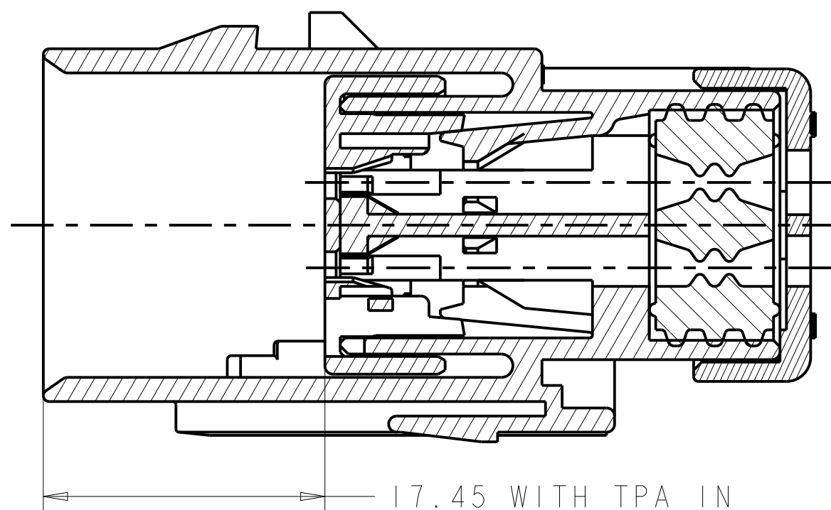
SECTION A-A
