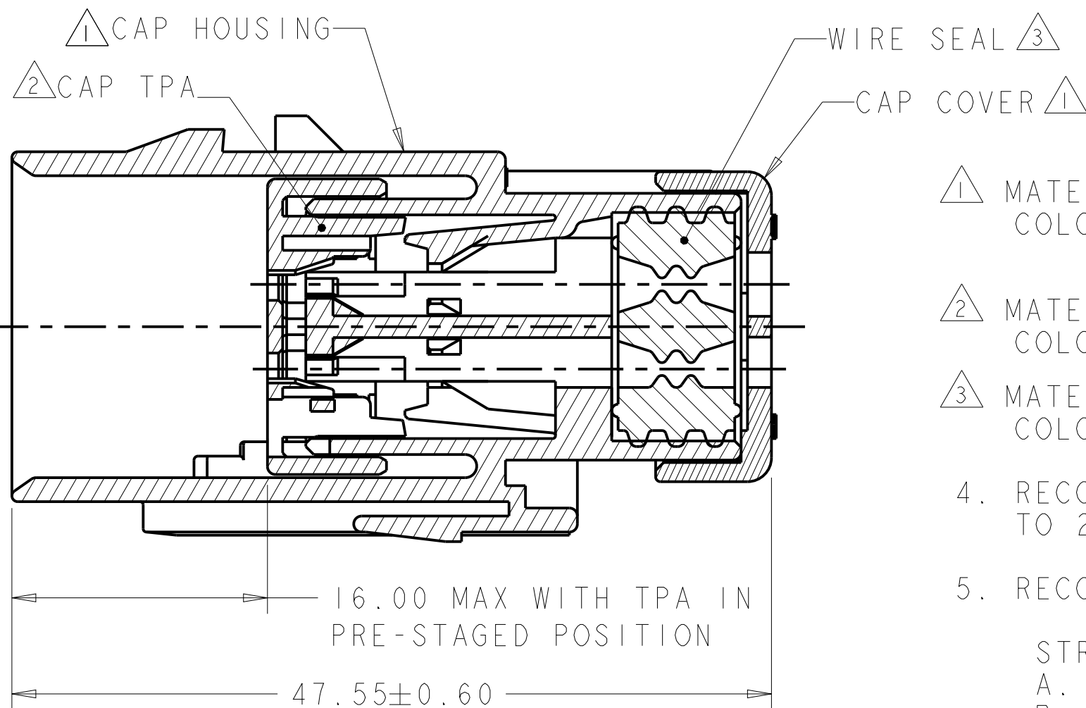
SECTION A-A
