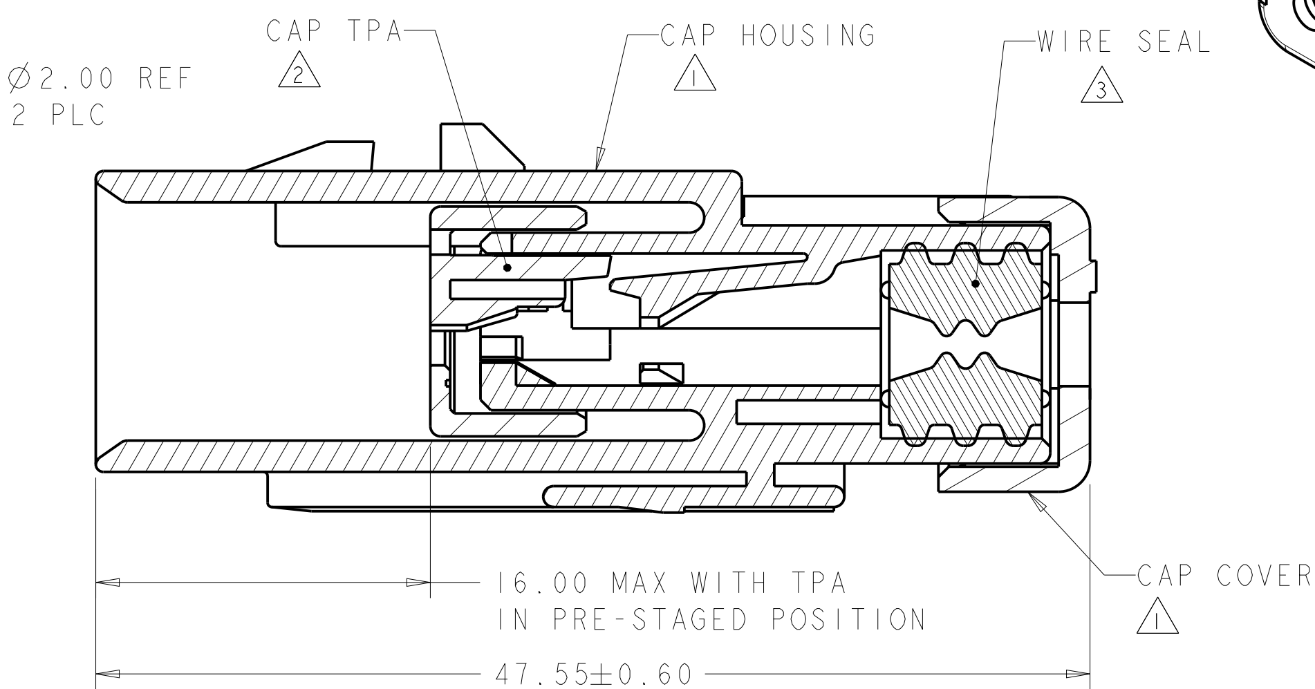
SECTION A-A
