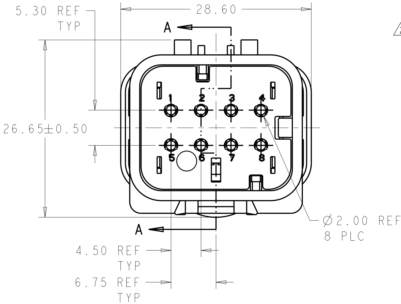
2320917-1 SHOWN KEY A
