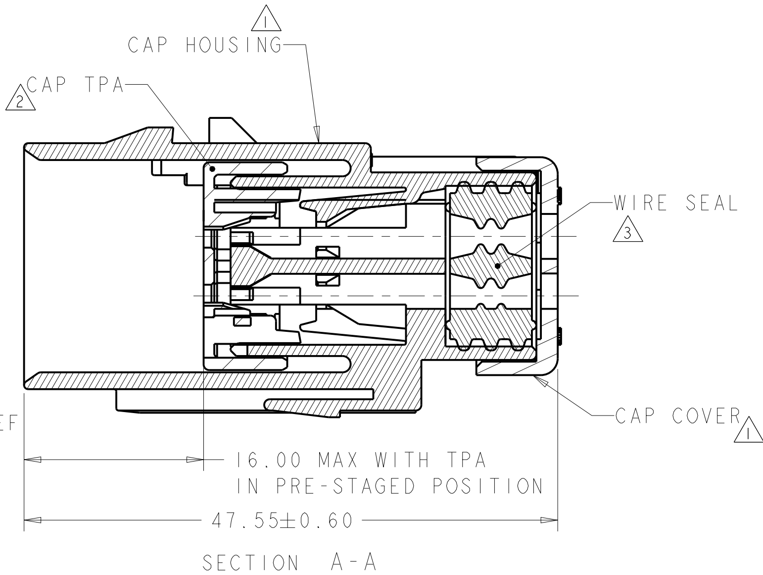
2320917-4 SCALE 2:1 KEY D
