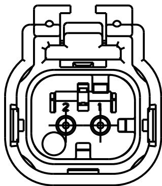
2320932-3 SCALE 2:1 KEY C
