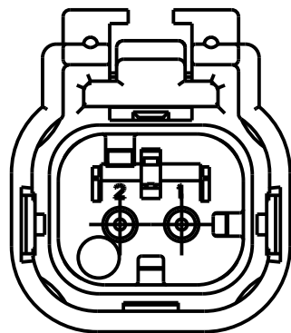
2320932-4 SCALE 2:1 KEY D
