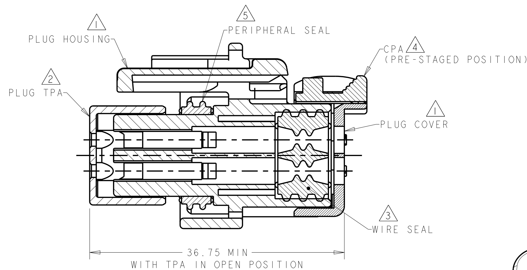
2320922-4 SCALE 2:1
