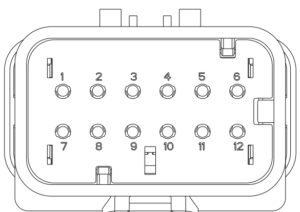
776438-3 SCALE 2:1
