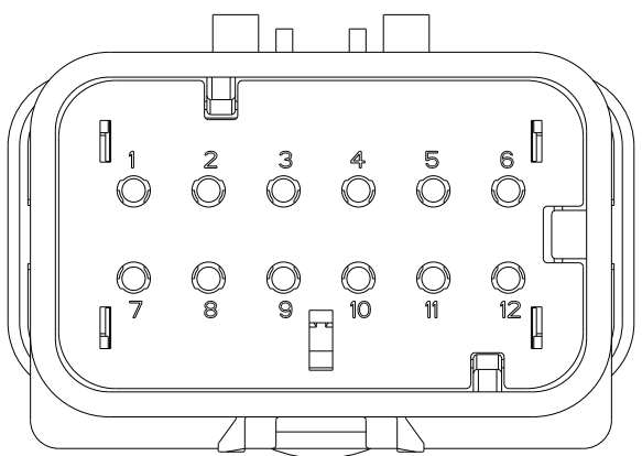
776438-2 SCALE 2:1
