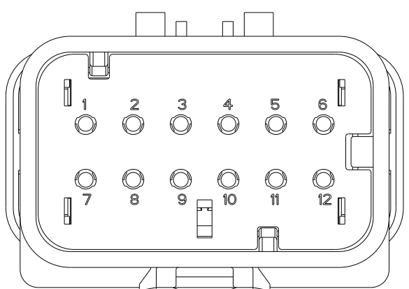
776438-4 SCALE 2:1
