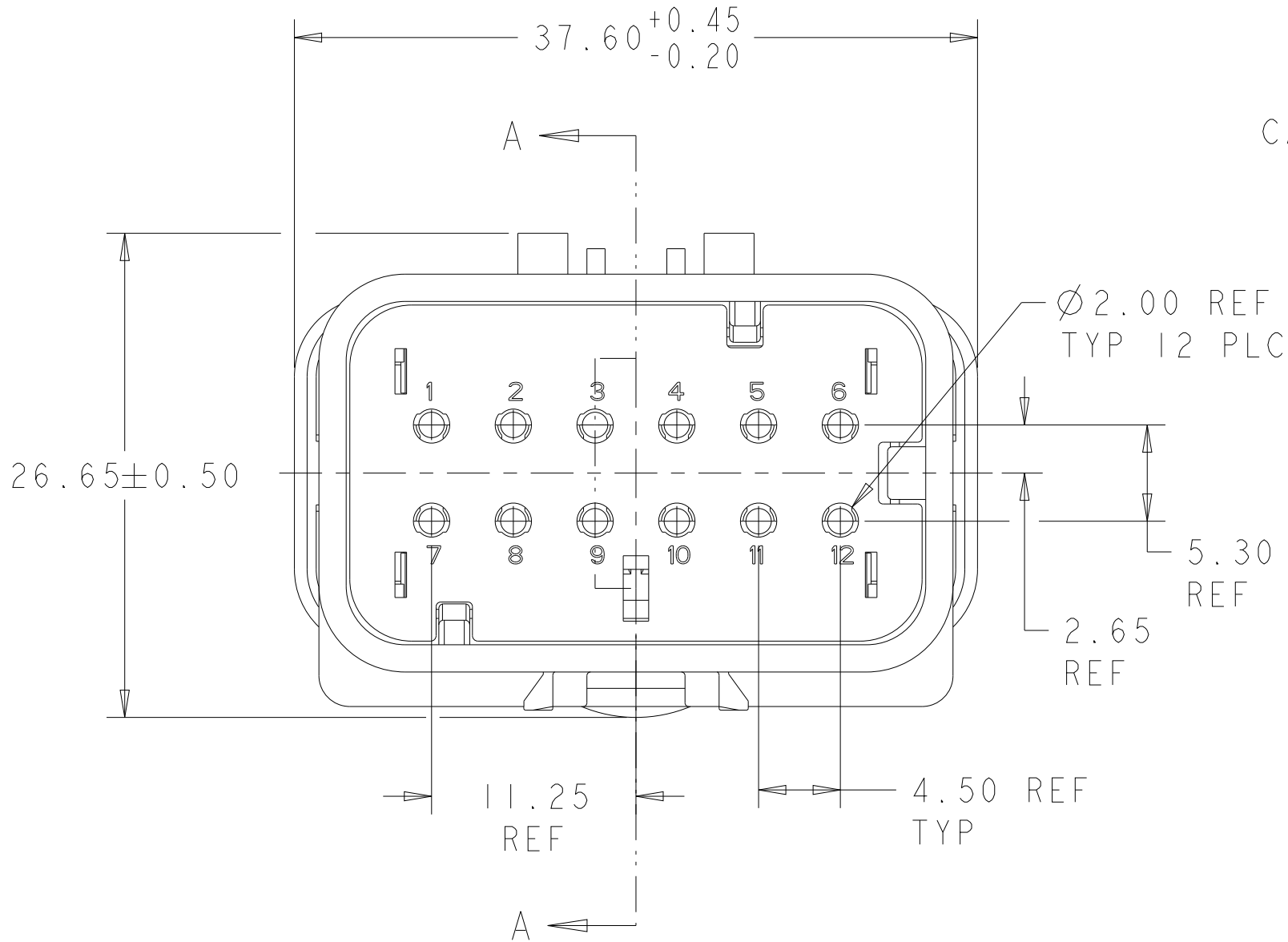
776438-1 SHOWN
