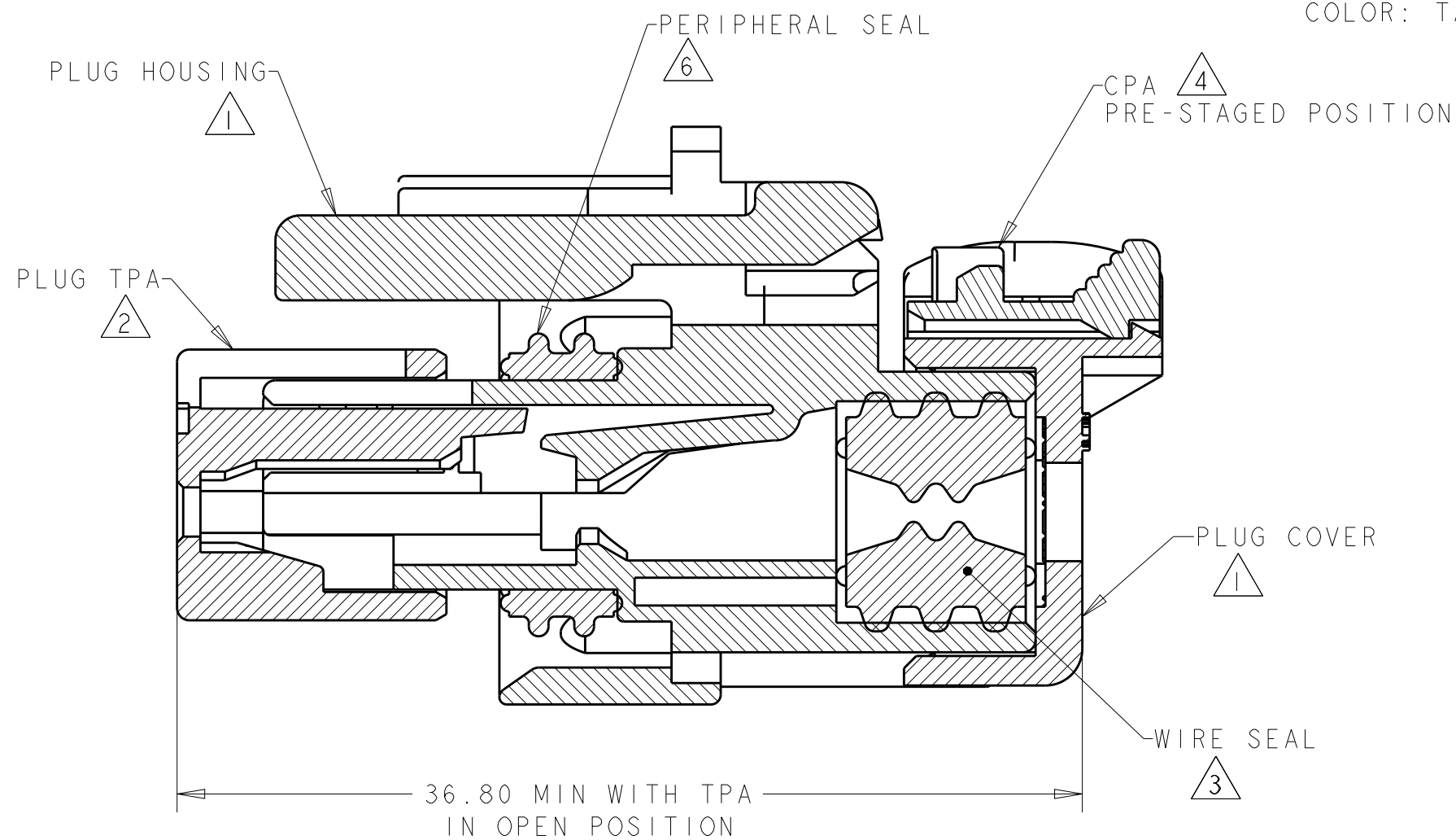
SECTION A-A
