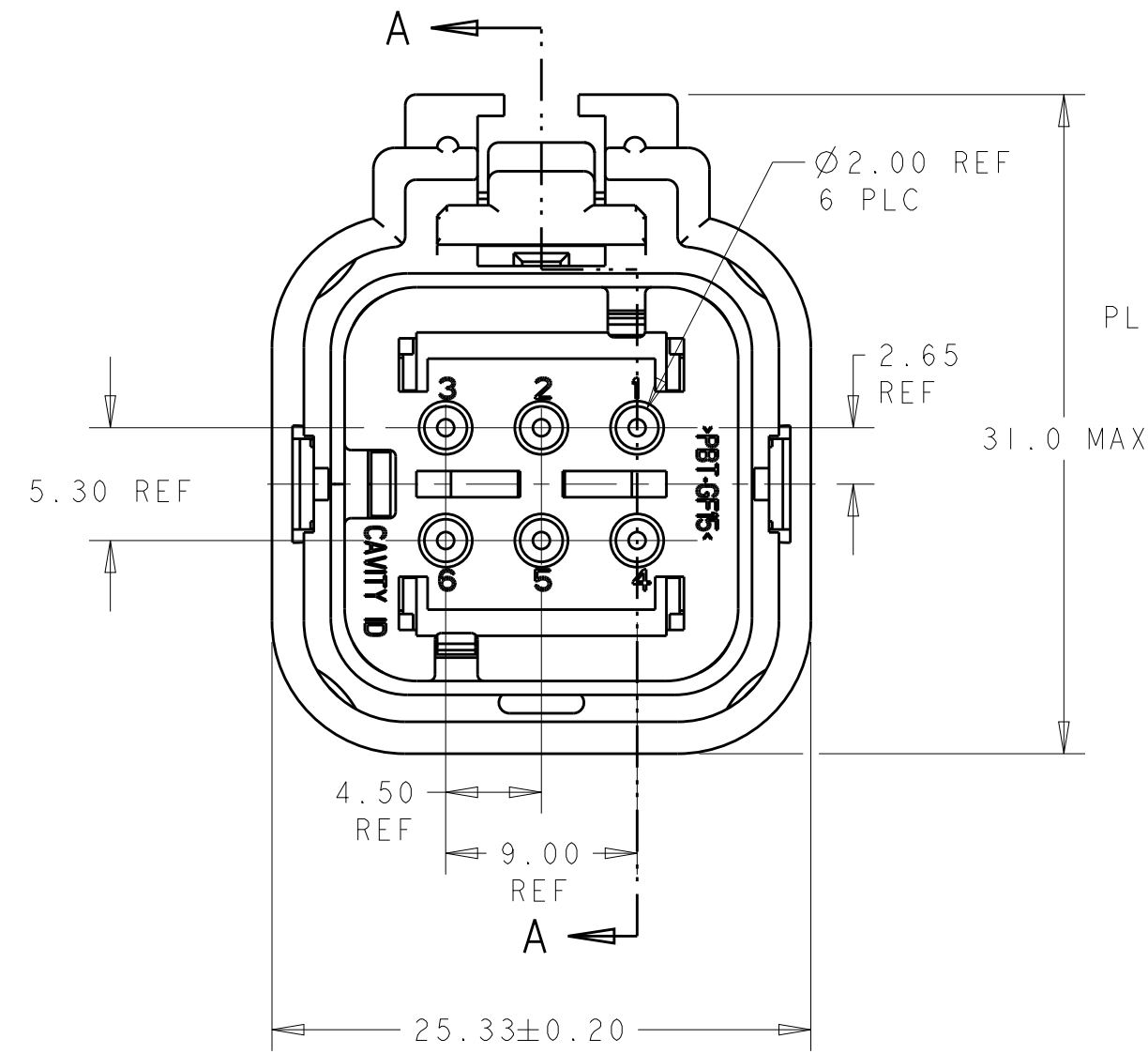
776531-1 SHOWN
