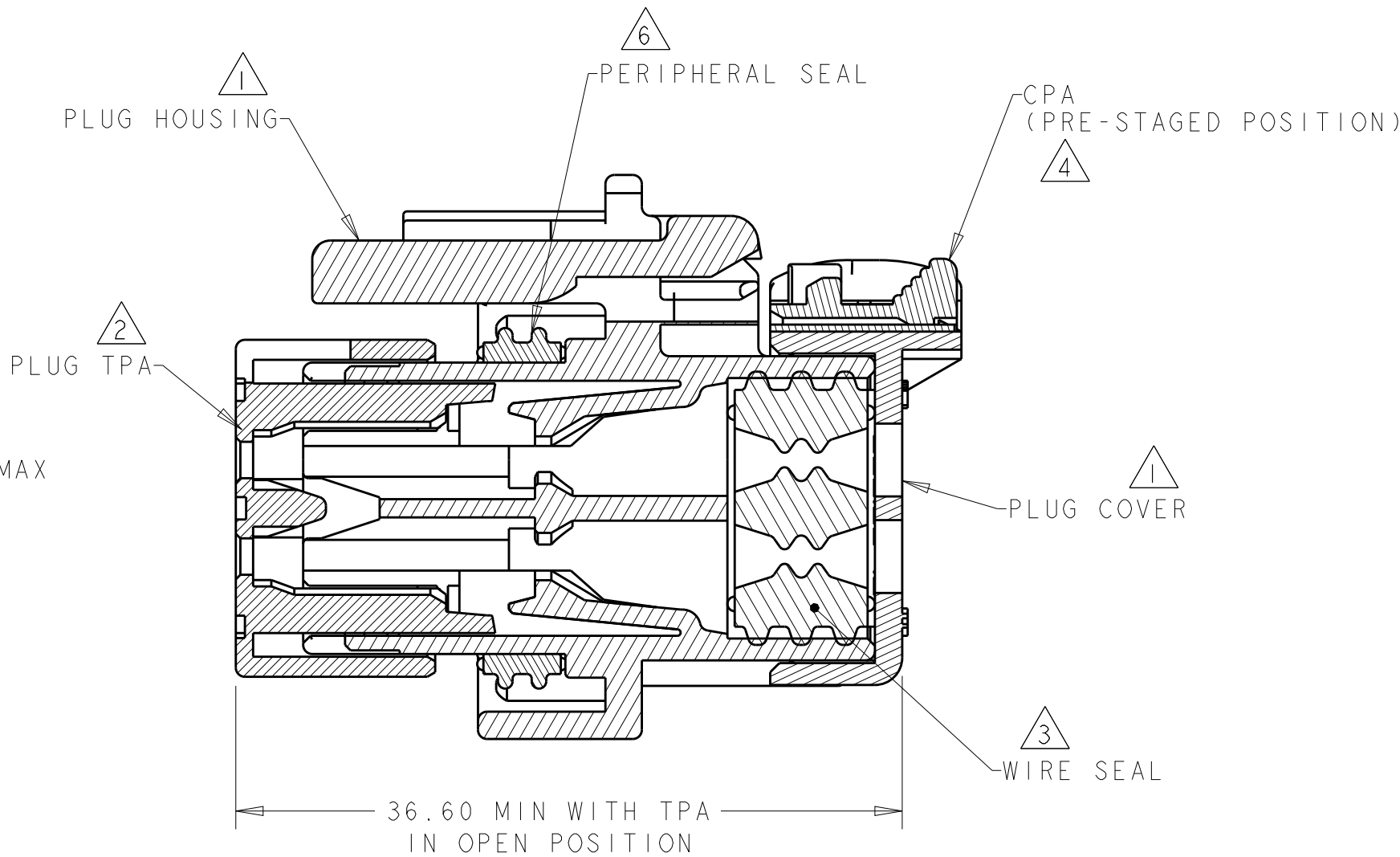
SECTION A-A
