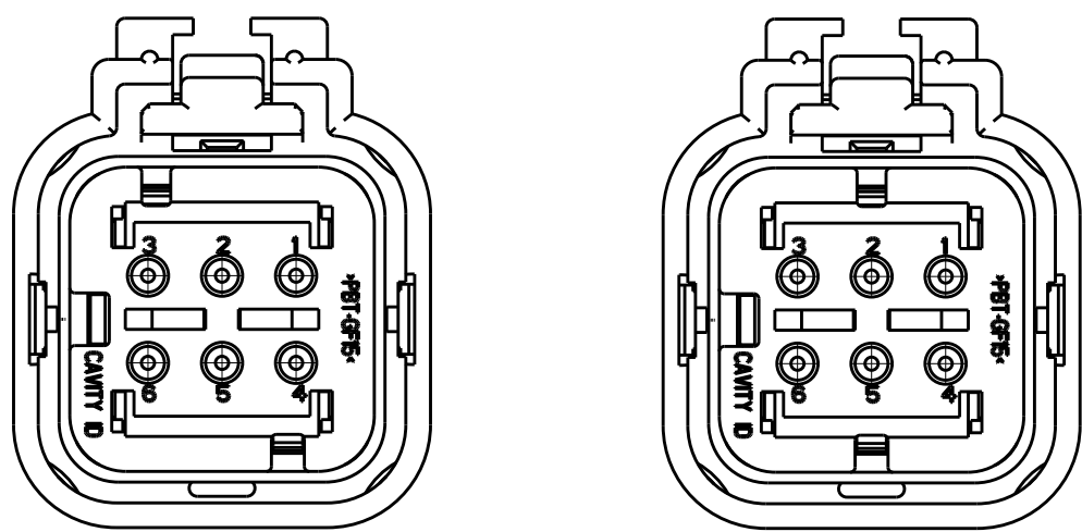
776531-2 SCALE 2:1
