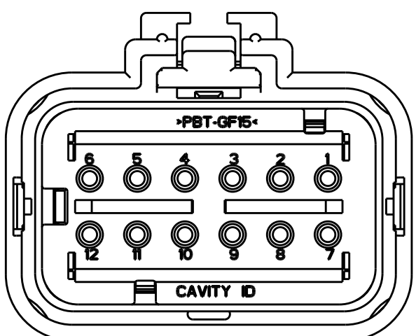
776437-4 SCALE 2:1
