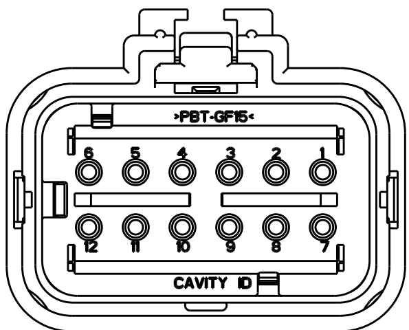
776437-3 SCALE 2:1
