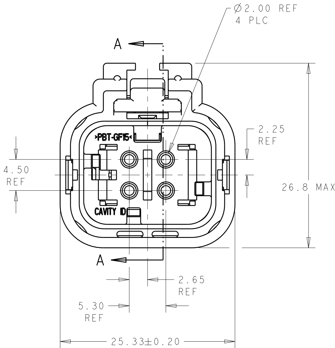
776487-1 SHOWN
