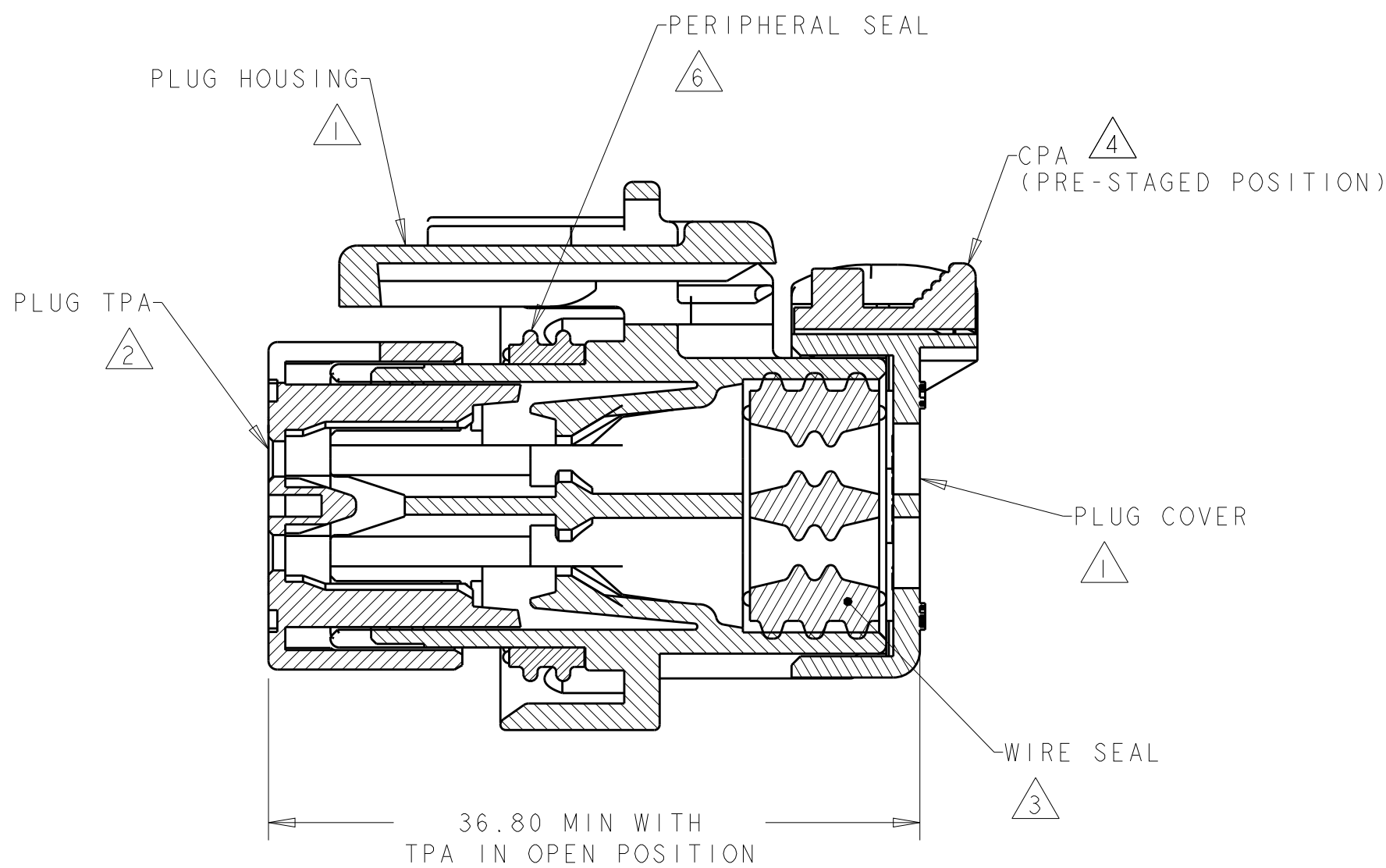
SECTION A-A
