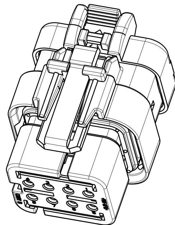
SCALE 2:1
