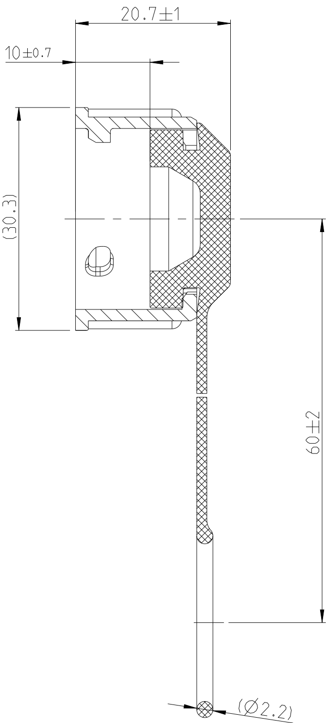
SECTION A-A
