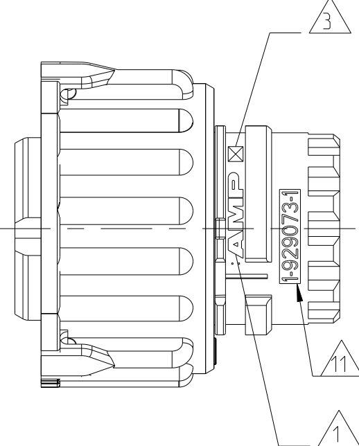
VIEW B ROTATED Ansicht B gedreht
