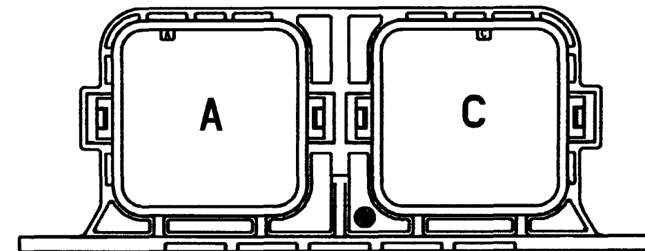
DRBF-3AC KEYS A & C
