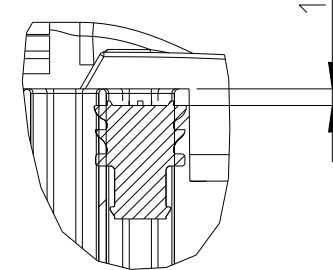
DETAIL "A" Einzelheit SCALE Maßstab
