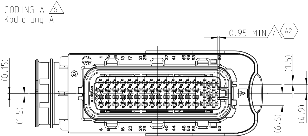
PRE LOCKED POSITION OF SECONDARY LOCKING Vorraststellung der 2. Kontaktsicherung
